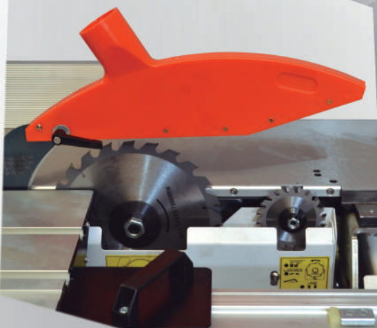
Grupo sierra e incisor Saw blade and scoring group Groupe disque et inciseur
